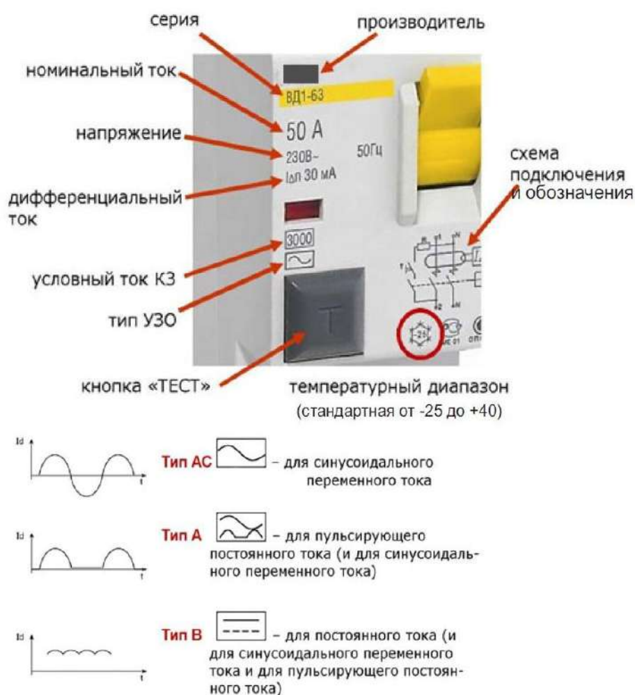
Рисунок 5. Маркировка УДТ
